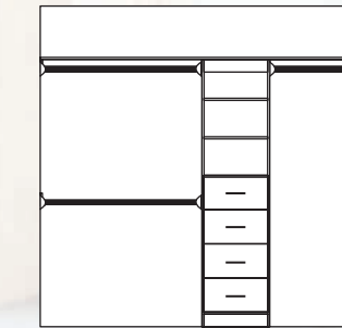
BIR 08A 2420mm Min Width 3680mm Max Width
