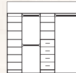
BIR 17A 3230mm Min Width 4800mm Max Width
