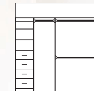
BIR 12A 3230mm Min Width 4800mm Max Width
