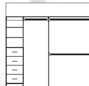
BIR 05B 1640mm Min Width 2460mm Max Width
