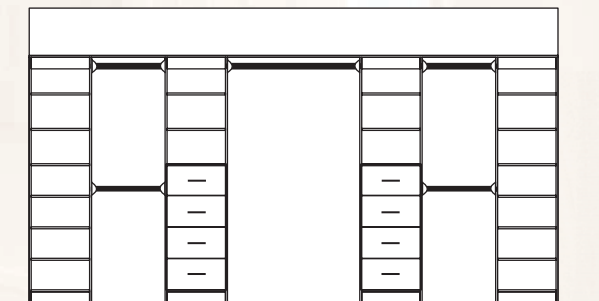
BIR 17A 3230mm Min Width 4800mm Max Width
