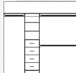
BIR 06A 1640mm Min Width 2460mm Max Width
