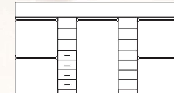
BIR 16A 2780mm Min Width 4800mm Max Width
