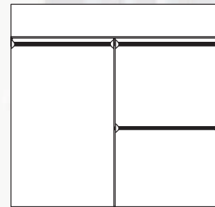
BIR 04A 800mm Min Width 2460mm Max Width
