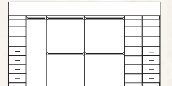
BIR 15B 3680mm Min Width 4800mm Max Width
